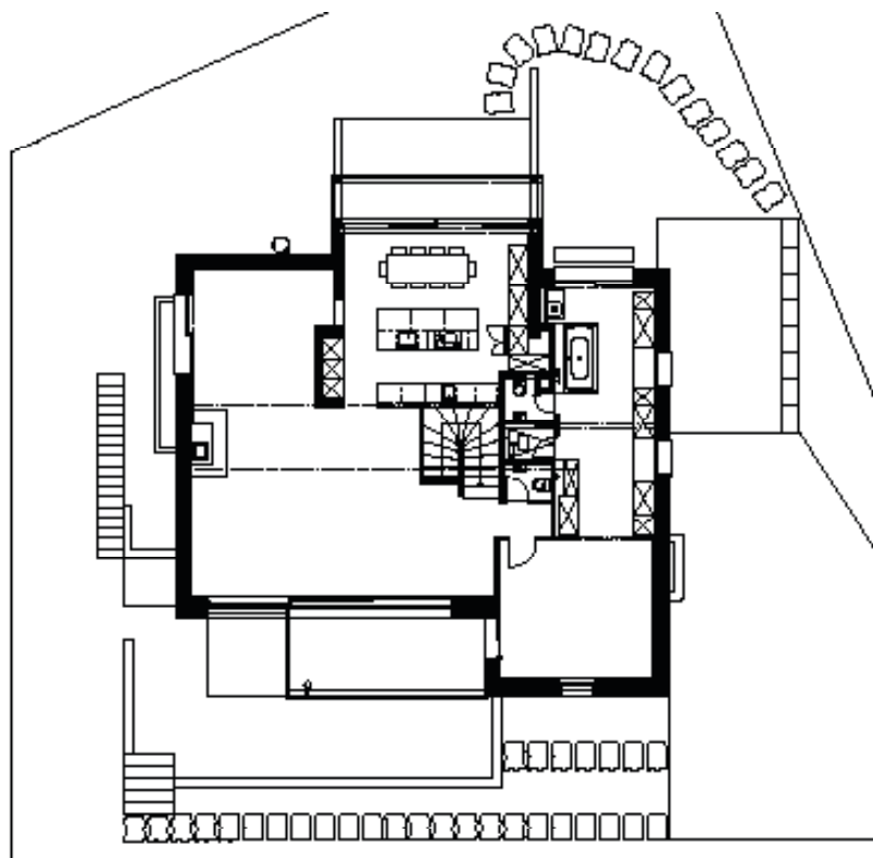
Erdgeschossplan
