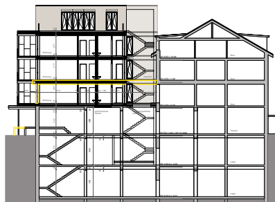
Erweiterung Güterstrasse 22 Bern Querschnitt Alt- und Neubau
