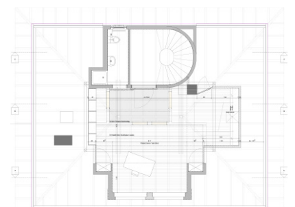
Mettlenhölzliweg 4 Muri Dachgeschoss Ausbau
