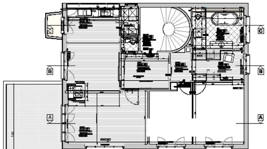
Erdgeschoss Wohnung Essbereich
