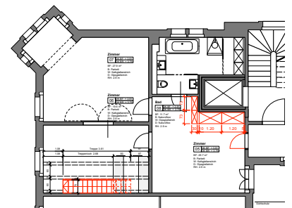
oben: Grundriss im Obergeschoss unten: Ansicht Treppe Erdgeschoss
