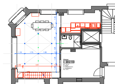
oben: Grundriss im Erdgeschoss unten: Ansicht Treppe im Erdgeschoss
