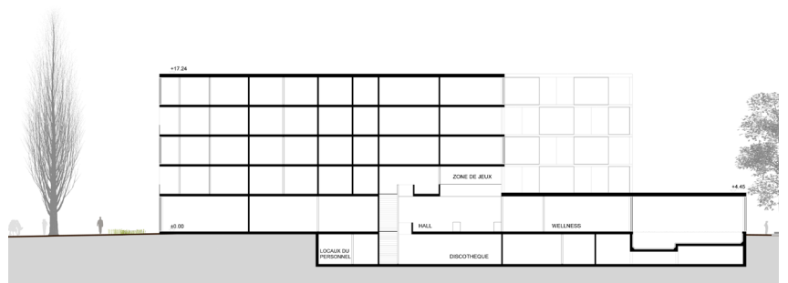
Coupe constructive Bâtiment
