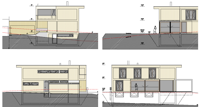
Einfamilienhaus Vorackerrain Gümligen Fassadenpläne
