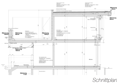
Schnittplan
