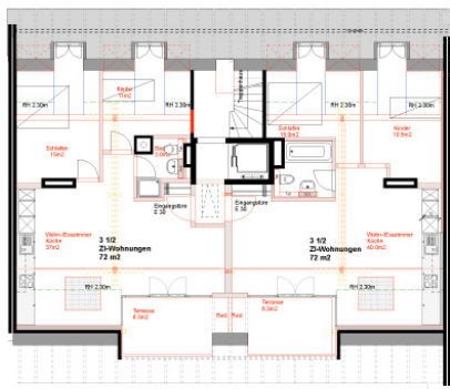
Grundriss zwei Dreizimmerwohnungen
