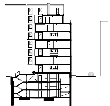
Immeuble locatif Rue Du-Bois-Melly Genève coupe de l'immeuble
