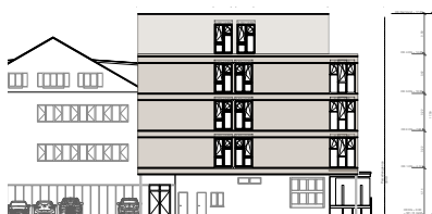
Erweiterung Güterstrasse 22 Bern Fassade Alt- und Neubau
